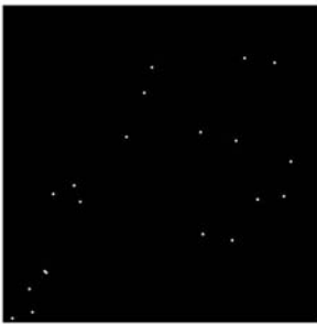
图 2 一幅投影模拟星图
