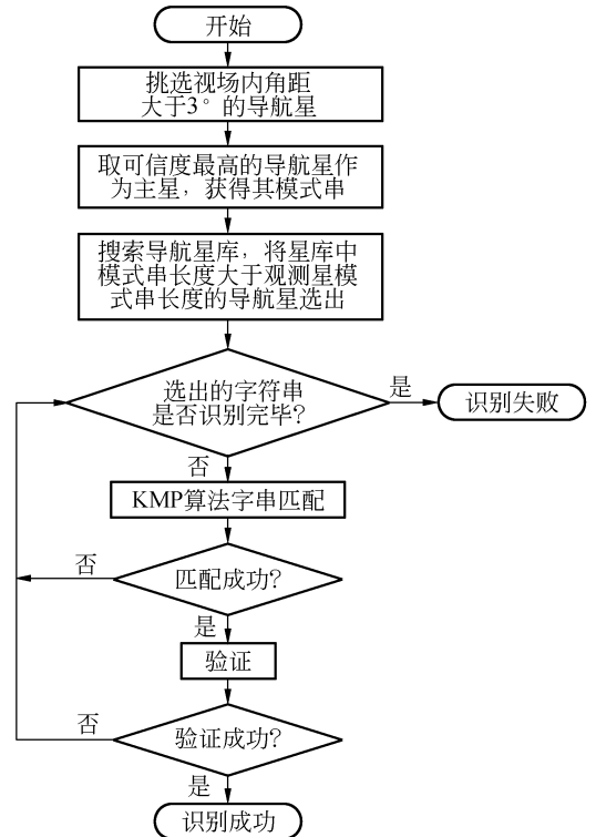
图 1 星图识别原理的流程图
