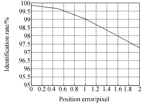
图 6 位置偏差对识别率的影响
