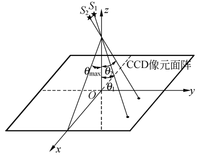
图 3 主星成像在 CCD 的中心 O
